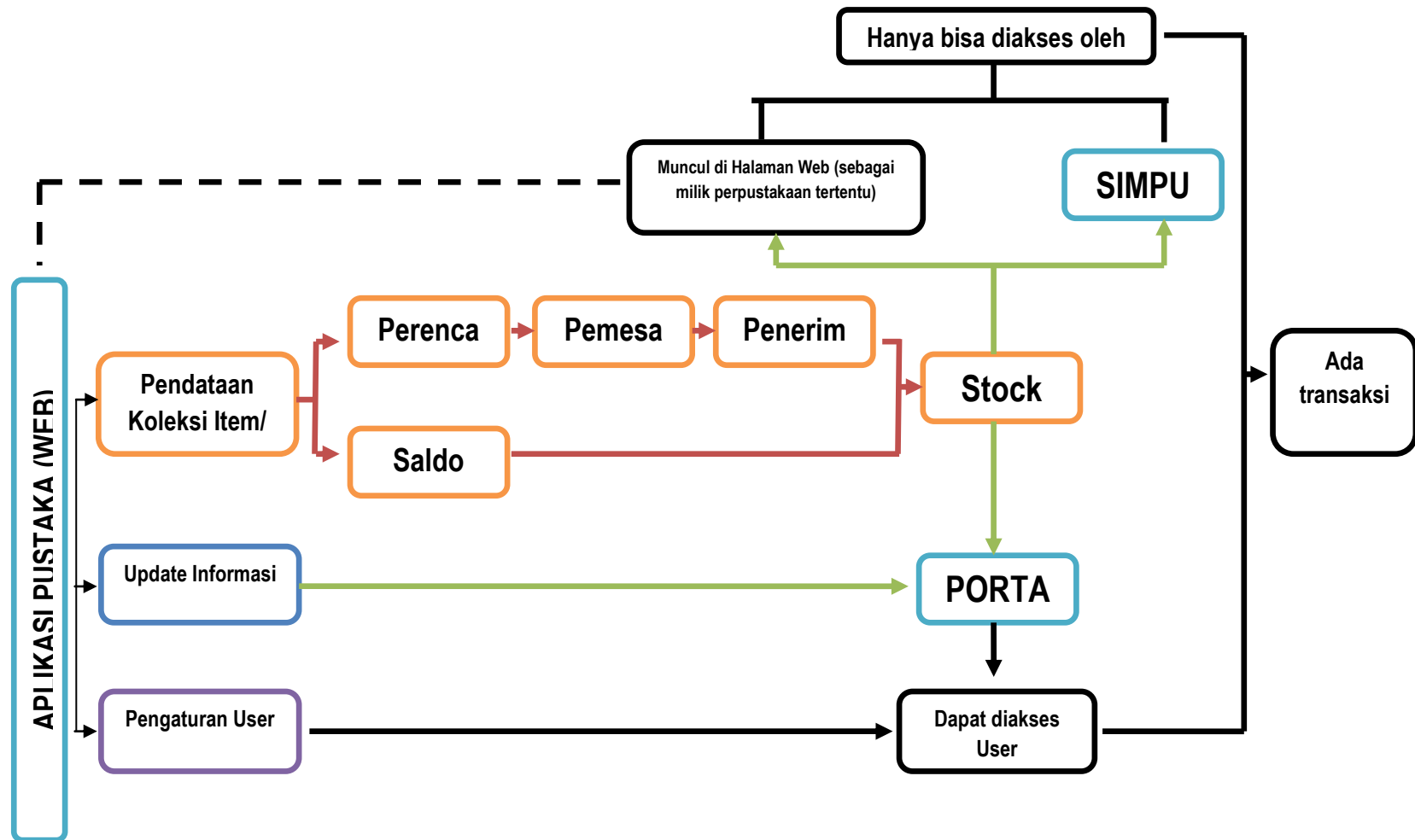
Alur Pengadaan Koleksi Perpustakaan – Transaksi Peminjaman/Pengembalian
